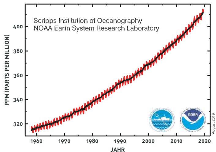
CO 2 -GEHALT DER ATMOSPHÄRE AM MAUNA LOA OBSERVATORIUM
